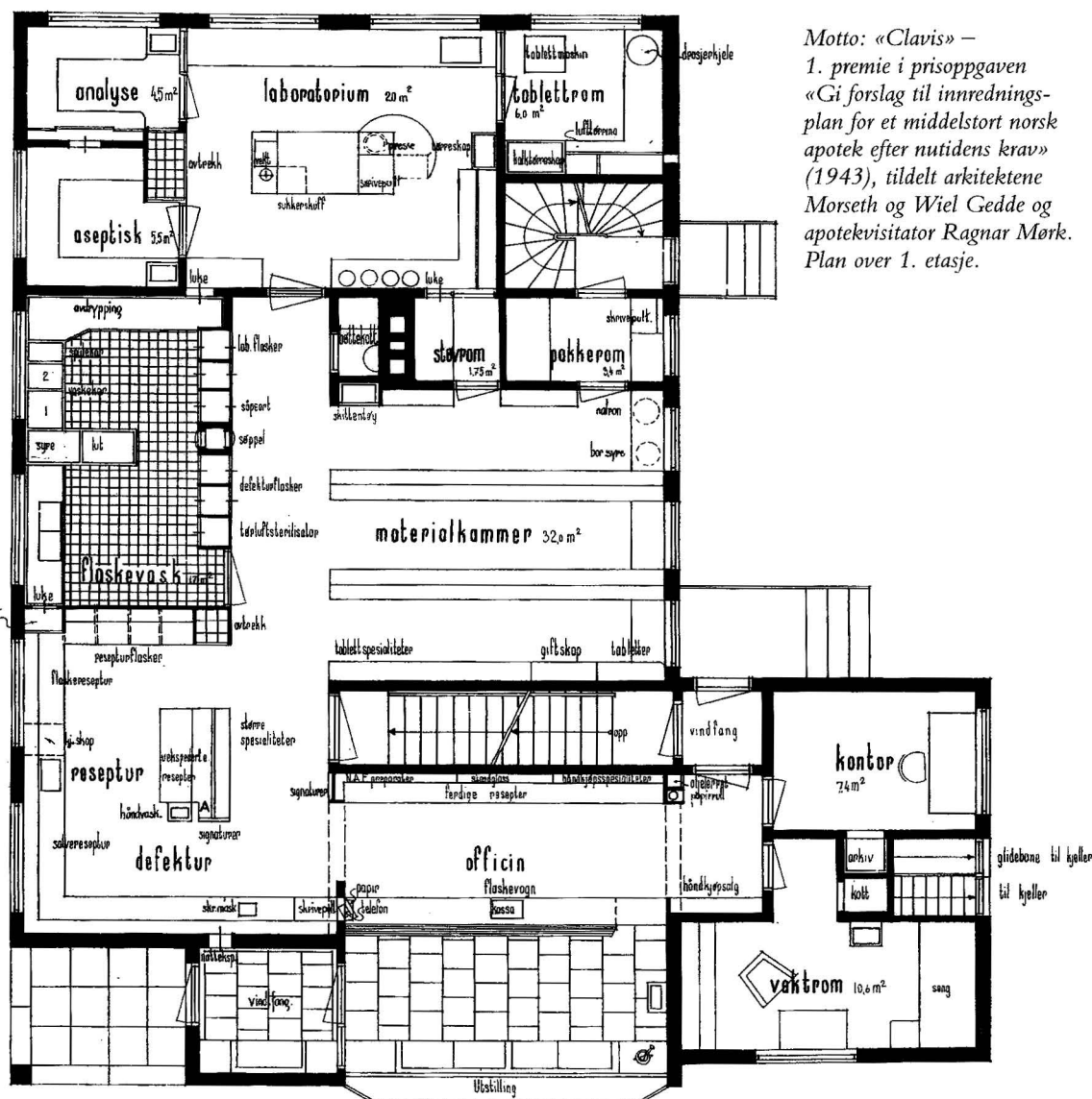
Plan over 1. etasje. 1:100
